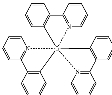
Ir(ppy) 3
