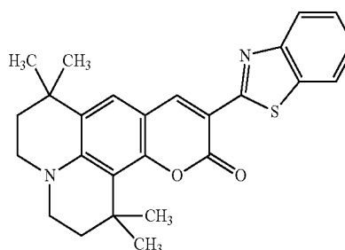
C545T
