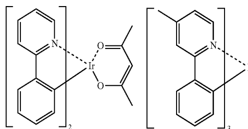
Ir(ppy) 2 (acac)
